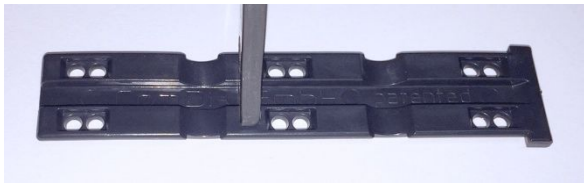
Abbildung 2: Gleitleiste SV35 – maximale Gegenbiegung (geradegebogen)
